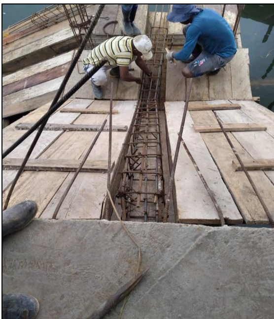
Foto 15: Armado de Escalera para su fundida Foto 16: escalera de muelle fundida
