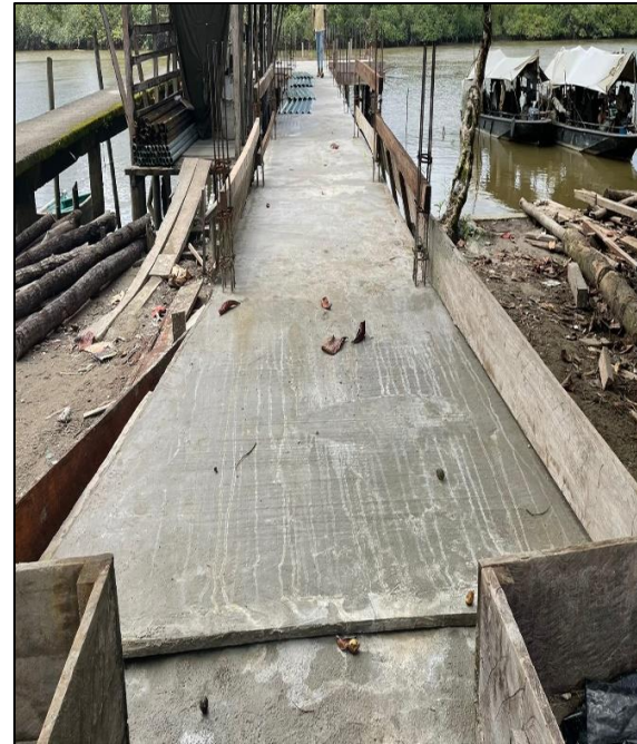
Foto 14: Placa de muelle fundida
