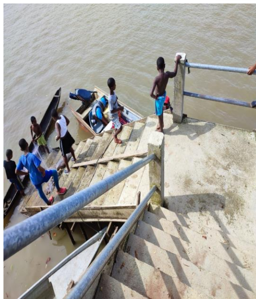
Foto 6: escalera de muelle Terminada
