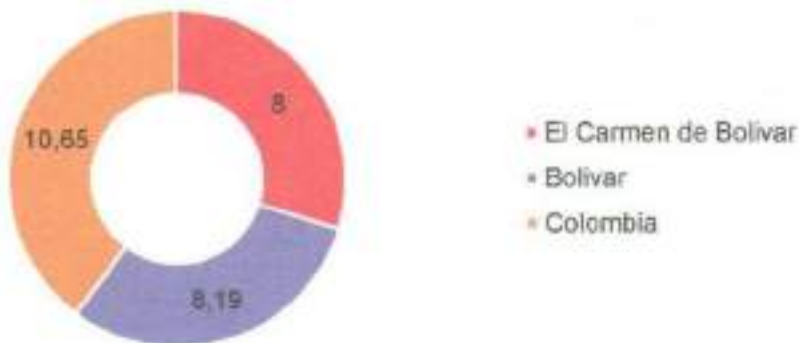
Figura 27. Rendimiento Yuca
