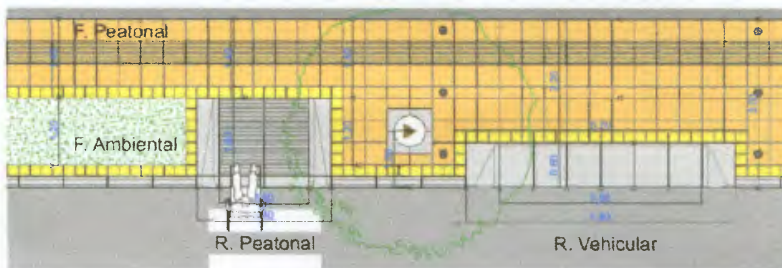
Gráfica N° 16. Rampas vehicular y peatonal en andenes de tres metros (3 m) en adelante.
