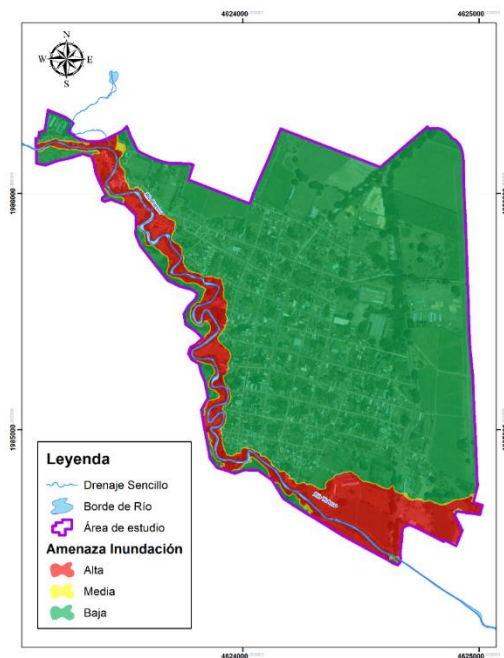
Mapa 15. Amenaza por inundación en la cabecera de Yotoco escala 1:5.000 Fuente: Consultoría, 2022
