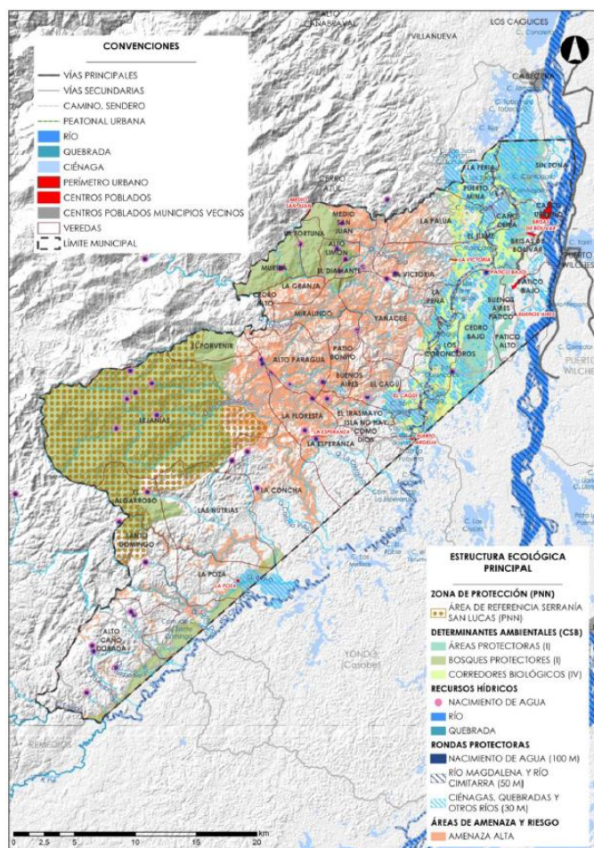
Ilustración 18. Estructura Ecológica Principal horizontal
