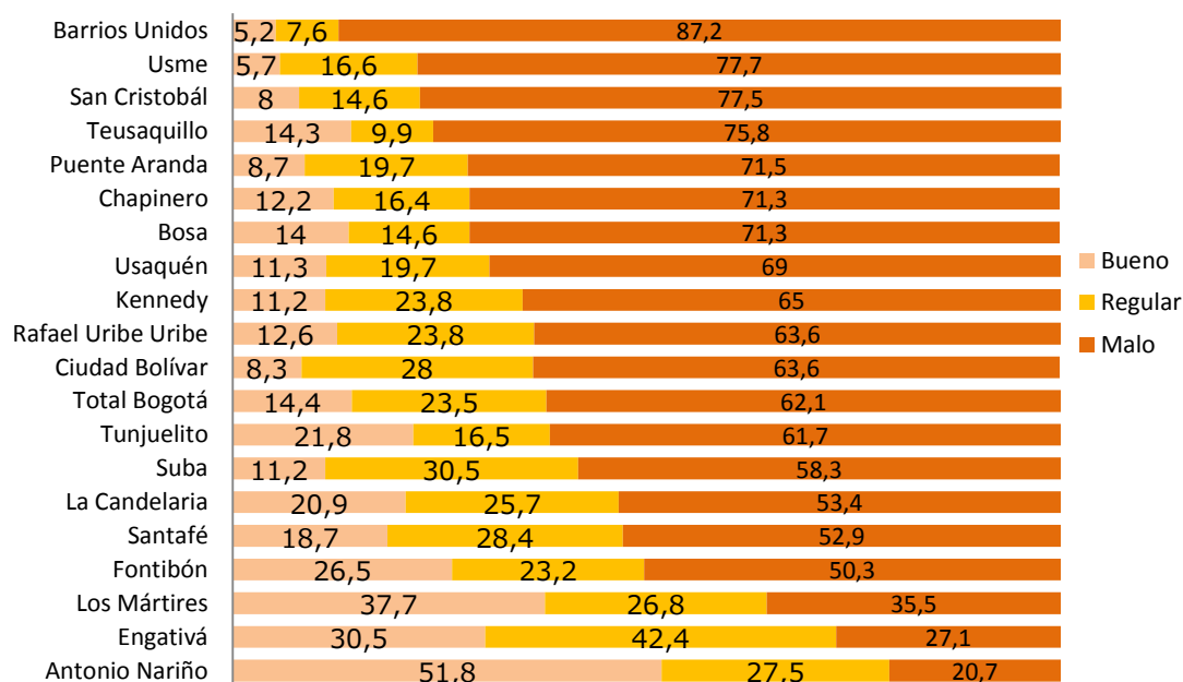
Gráfica No. 58 Inventario y diagnóstico de la malla vial local año 2011
