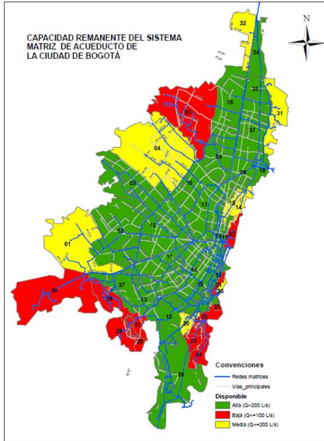
ILUSTRACIÓN 71 - CAPACIDAD REMANENTE DEL SISTEMA MATRIZ DE ACUEDUCTO DE LA CIUDAD DE BOGOTÁ. FUENTE PMMA EAB ESP 2016-2025.
