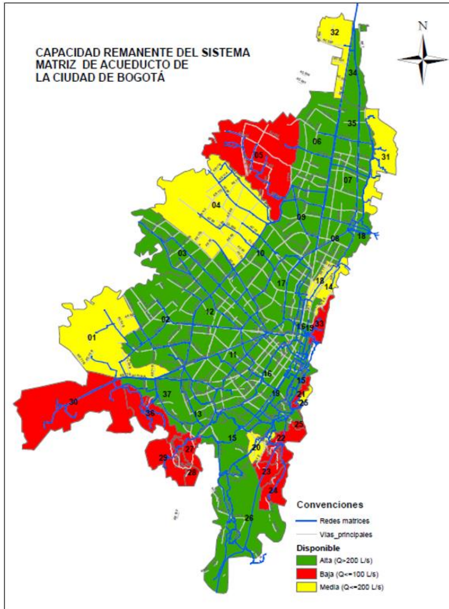
ILUSTRACIÓN 88 - CAPACIDAD REMANENTE DEL SISTEMA MATRIZ DE ACUEDUCTO DE LA CIUDAD DE BOGOTÁ. FUENTE PMMA EAB ESP 2016-2025.
