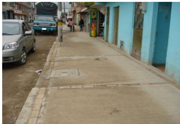
PAVIMENTO RÍGIDO ANDENES BARRIO EL SOSIEGO
