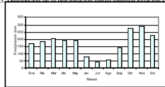
Figura 3. Distribución de la precipitación media mensual Estación La Fonda - Citec.
