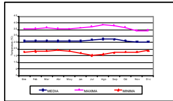
Figura 5. Distribución de la temperatura. Estación La Fonda Citec.
