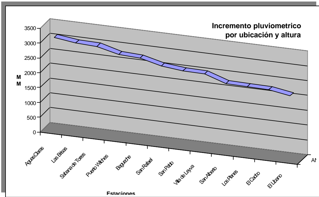
Figura 4. Tendencia de precipitación anual
