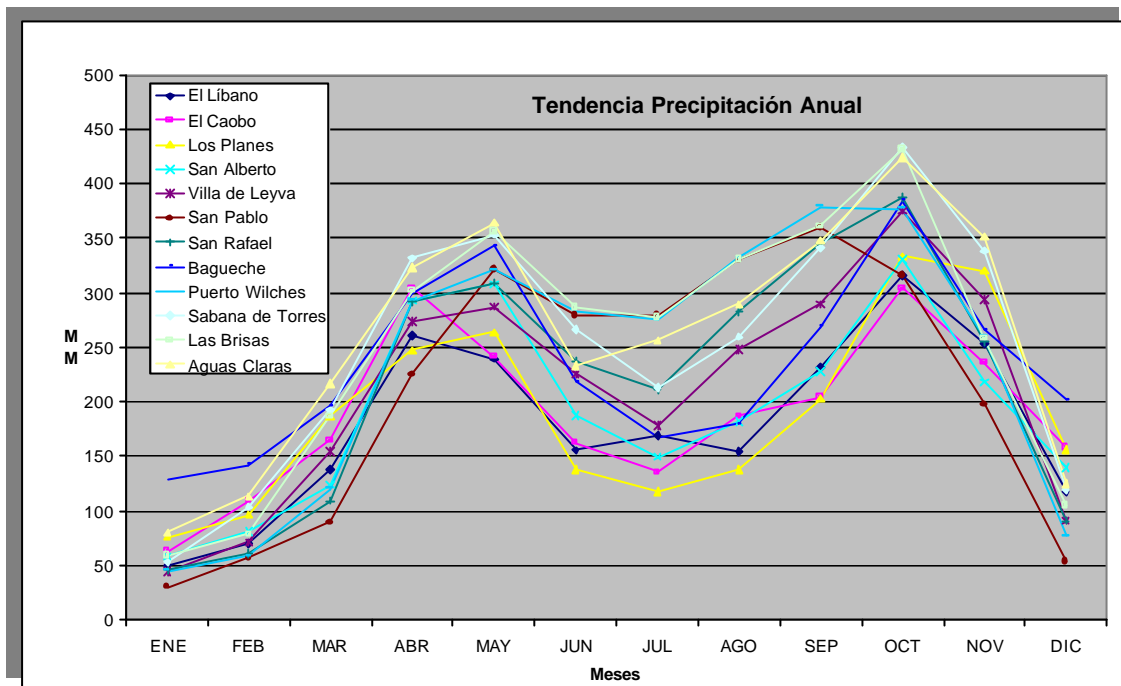
Figura 5. Incremento pluviométrico por ubicación y altura
